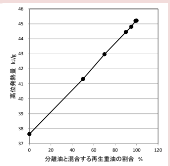
高位発熱量の変化
