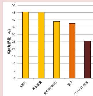
高位発熱量の比較
