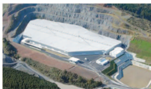
マルチバリアコンセプトに基づく被覆型処分場
