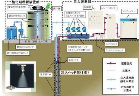
酸化剤の霧状酸化剤散布による環境修復 (ジェイ環境、ジェーハック)
