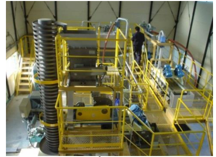
廃棄物洗浄分級プラント (韓国現代建設)
